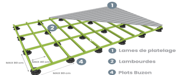
Double structure en lambourdes
